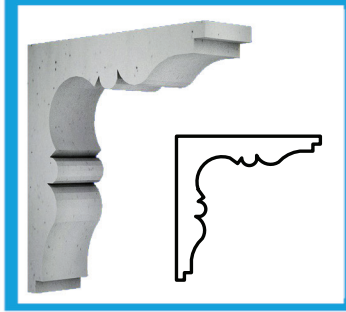
PY 3 50 x 50 x 15 cm
