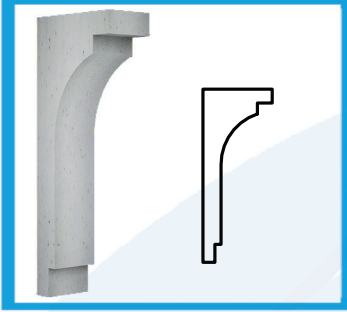
PY 5 50 x 20 x 15 cm
